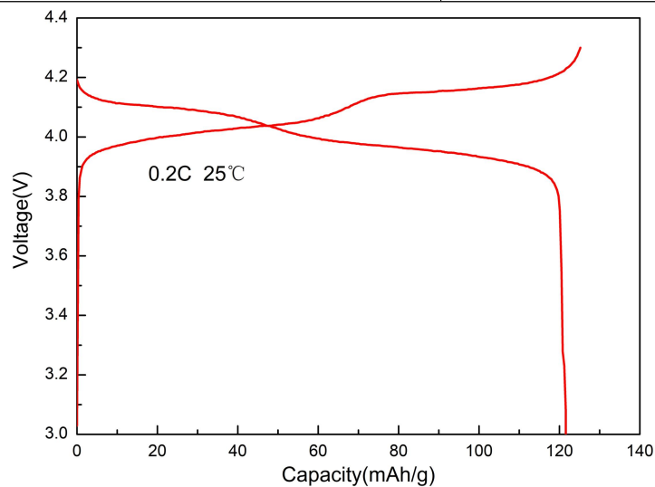
DXM-1181B 充放电曲线
