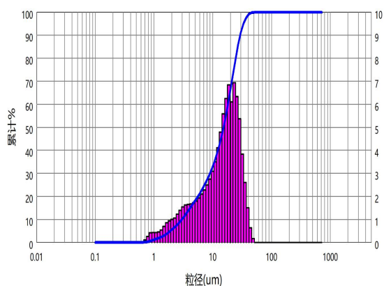
DXM-1181B 激光粒度分布曲线
