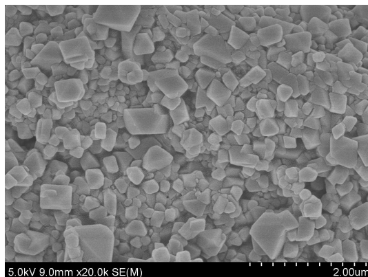
DXM-1181A SEM
