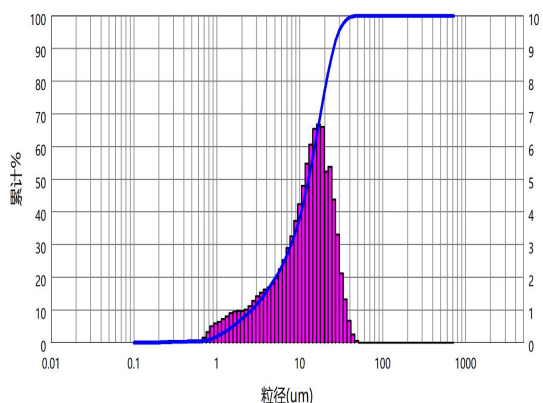
DXM-1181A 激光粒度分布曲线
