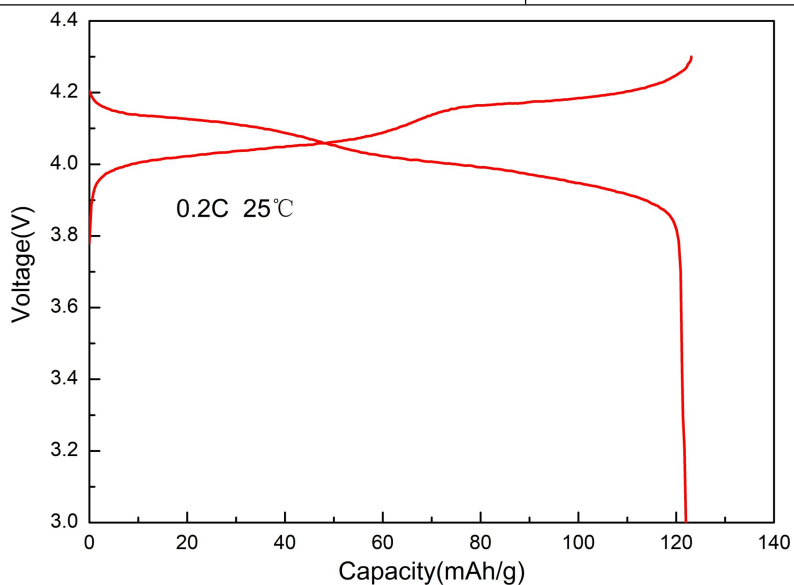
DXM-1181A 充放电曲线
