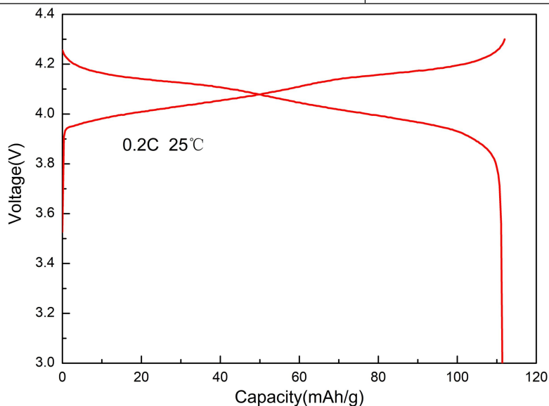
DXM-1182G 充放电曲线
