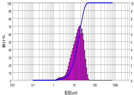
DXM-1182G 激光粒度分布曲线
