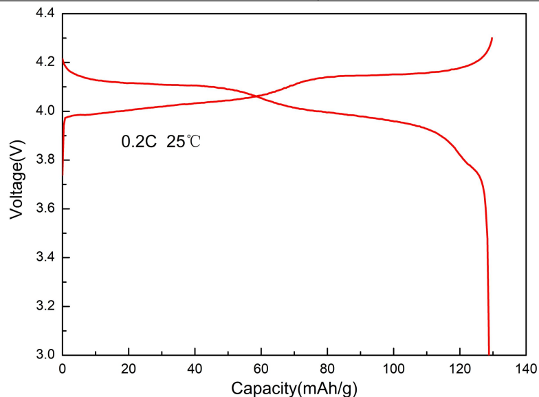
DXM-125 充放电曲线
