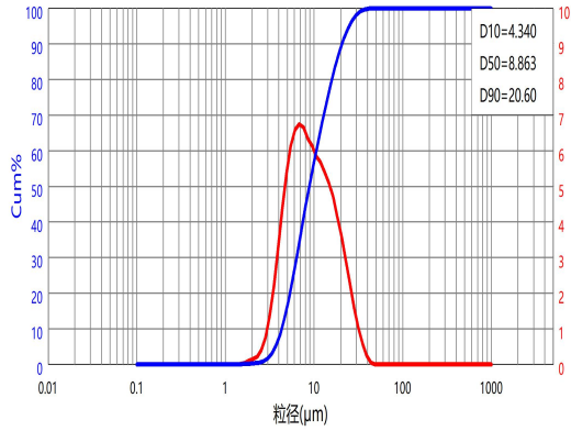
DXM-125 激光粒度分布曲线
