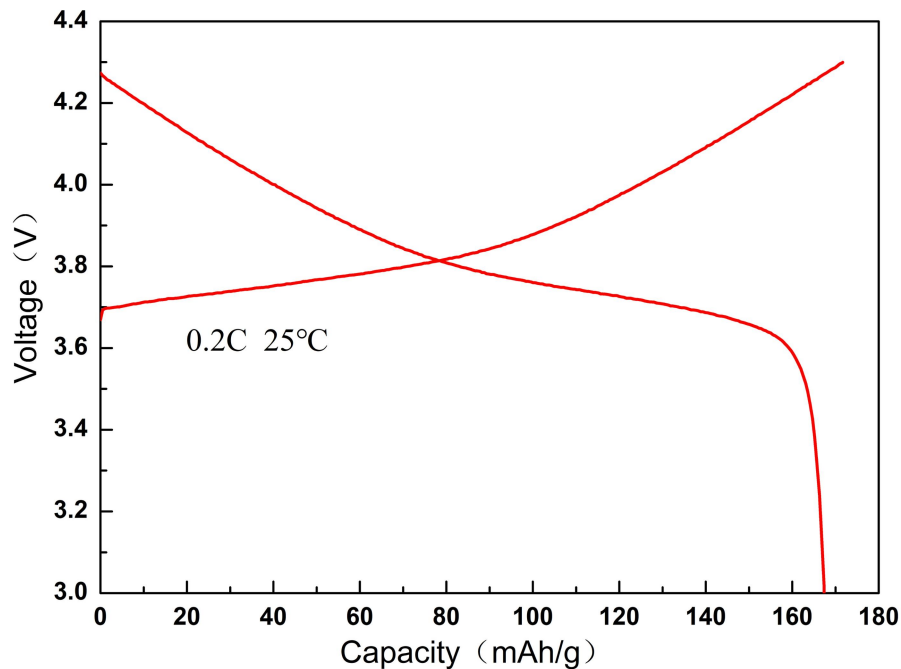
DXN-55 充放电曲线
