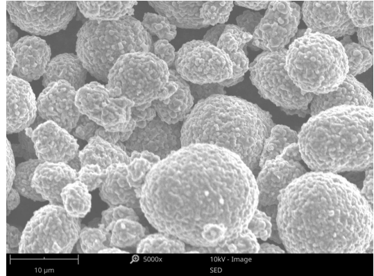
DXN-55 SEM
